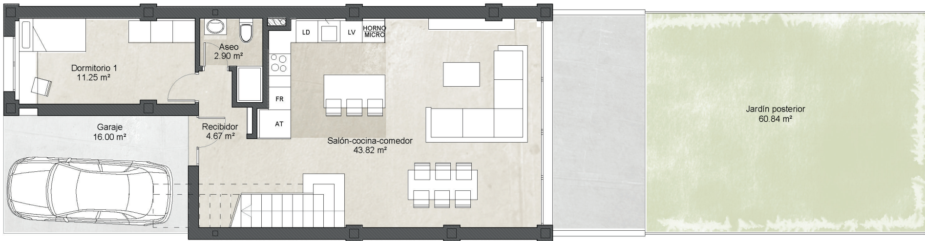
PLANTA BAJA
