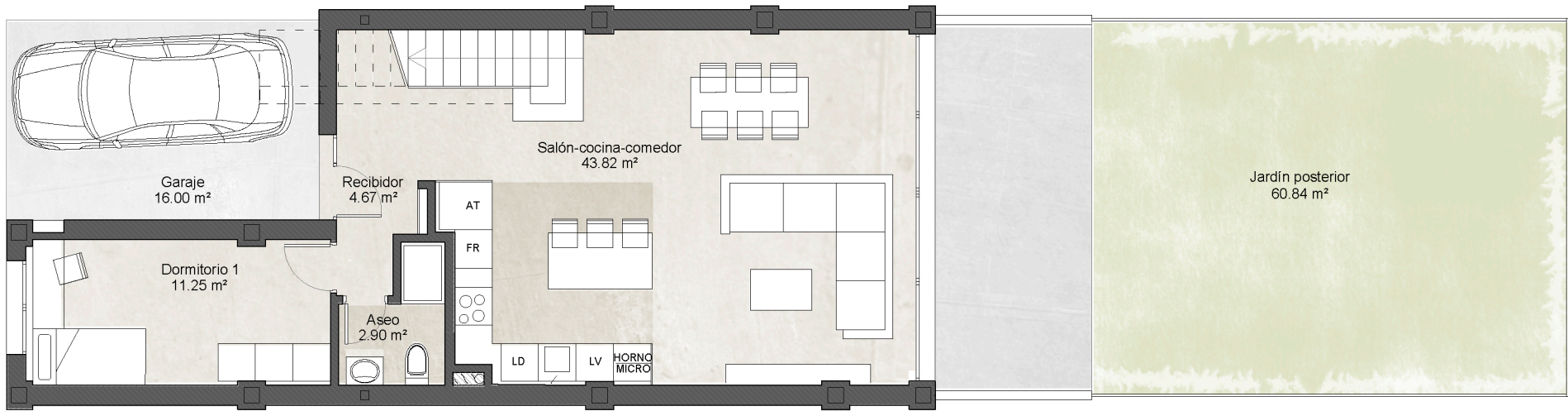
PLANTA BAJA
