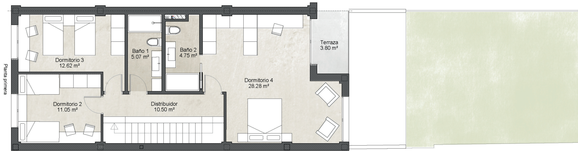
PLANTA PRIMERA
