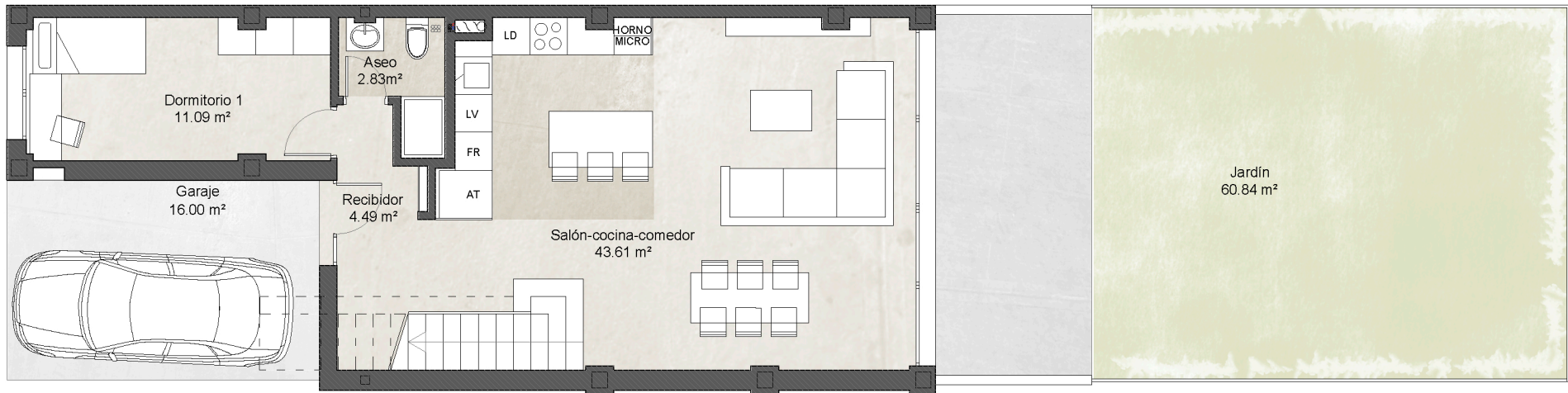
PLANTA BAJA
