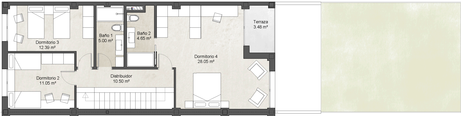
PLANTA PRIMERA
